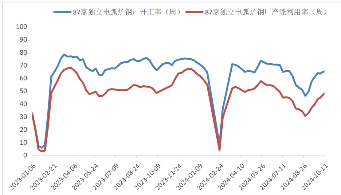
图3 全国独立电弧炉生产情况统计
